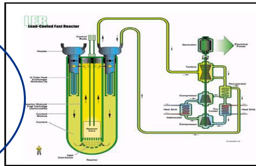
Réacteur rapide au Plomb
