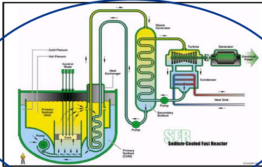
Réacteur rapide au Sodium
