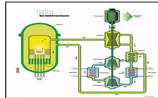
Réacteur rapide à gaz
