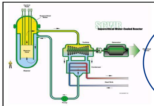
Réacteur à eau supercritique
