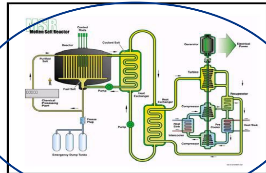
Réacteur à sels fondus
