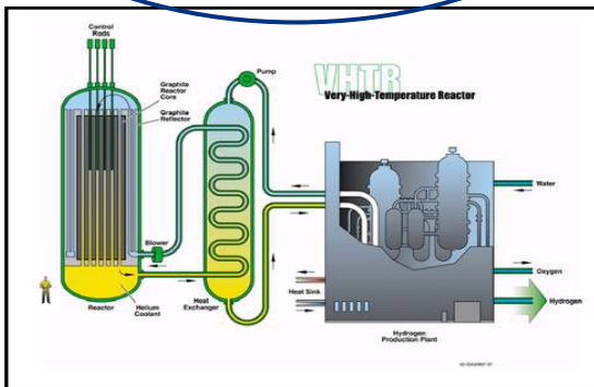
Réacteur à gaz, Très Haute Température
