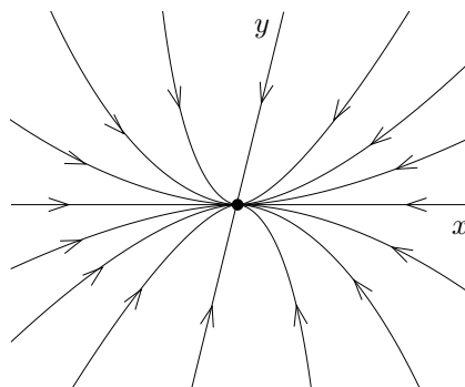
\lambda_2 < \lambda_1 < 0 nœud impropre stable
