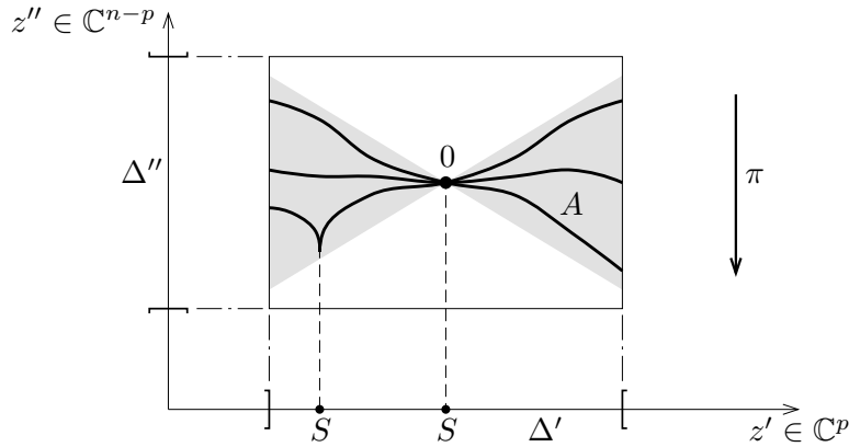
Fig. 2. Revêtement ramifié de A sur \Delta' \subset \mathbb{C}^p .
