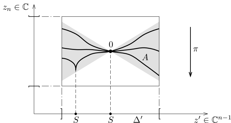
Fig. 1. Revêtement ramifié de A sur \Delta' \subset \mathbb{C}^{n-1} .
