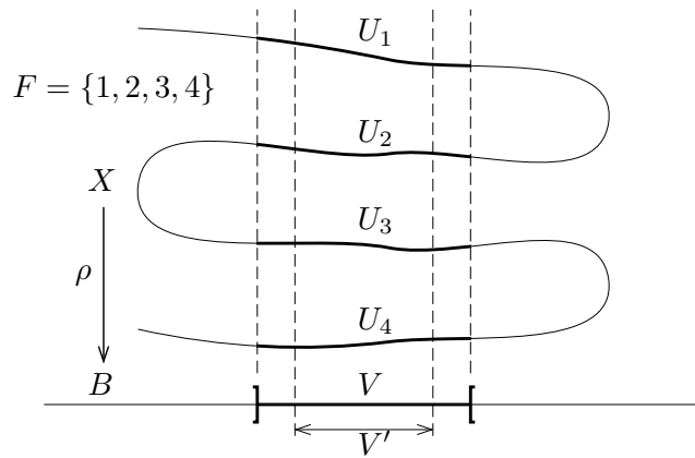
Fig. 3. Revêtement \rho : X \rightarrow B de fibre F .
